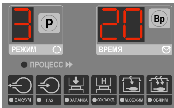
Рисунок 2.3 - Расположение таймера и индикаторов панели управления
