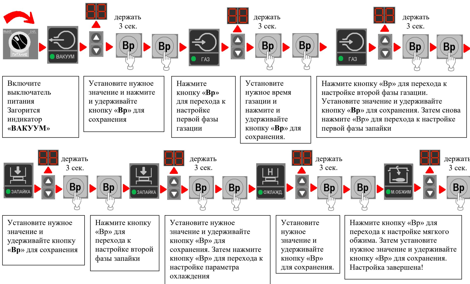
Рис. 2.6 – Порядок настройки параметров одного режима
